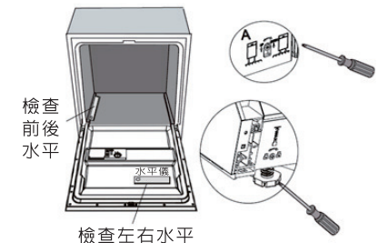
【圖8】腳調整圖示 註：腳的最大調整行程是50mm
