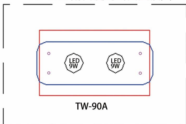
TW-90A 陽台使用所占面積圖
