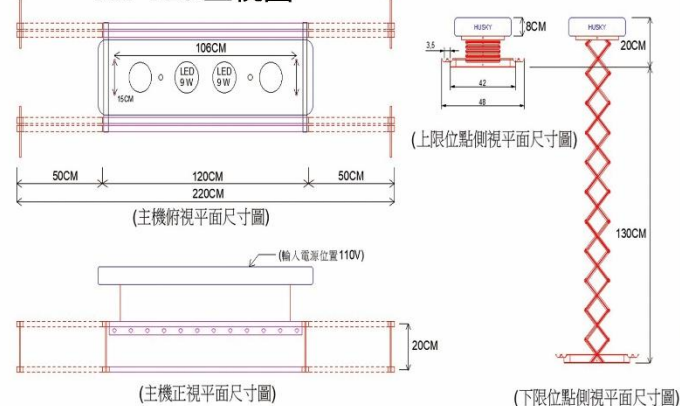
TW-120 三視圖
