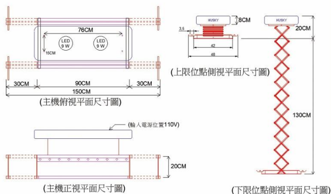
TW-90A 上下升降左右伸縮圖
