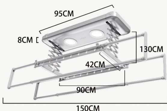
規格圖
