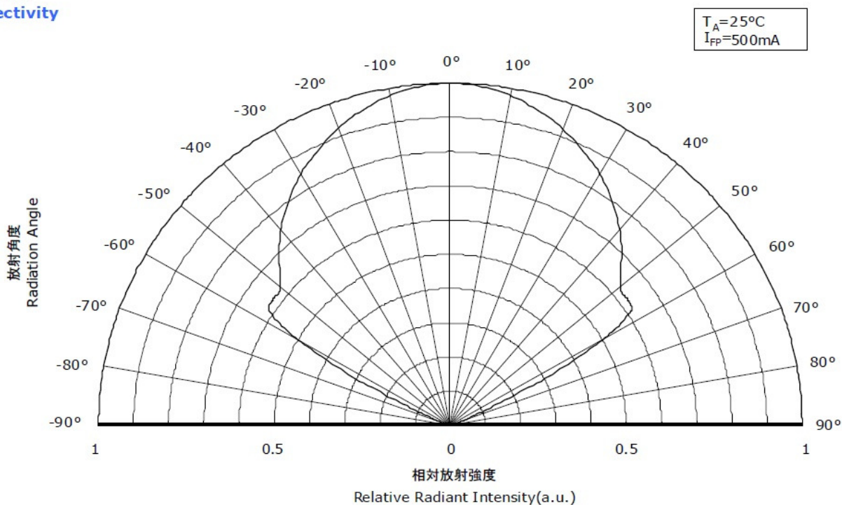
指向特性 Directivity
