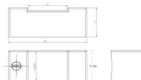
ALA-T53 外形尺寸圖
