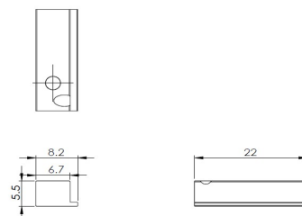
ALA-T63 外形尺寸圖
