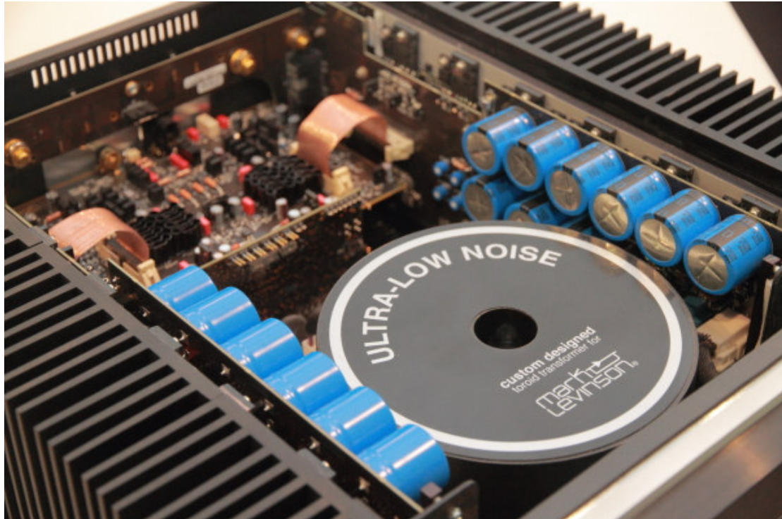
No. 536 的線路佈局，乾淨又工整，確實是有潔癖的設計工程。
