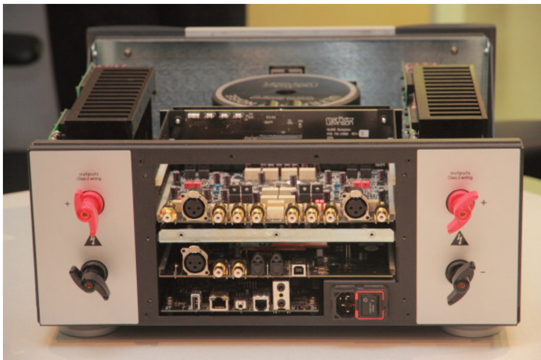
No. 585 綜合擴大機拆開來的模樣。
